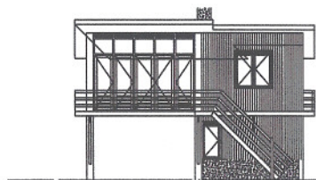
VOORGEVEL
