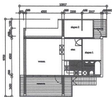
WONING 3000+
